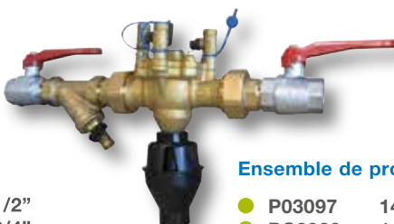
Disconnecteurs BA2860
