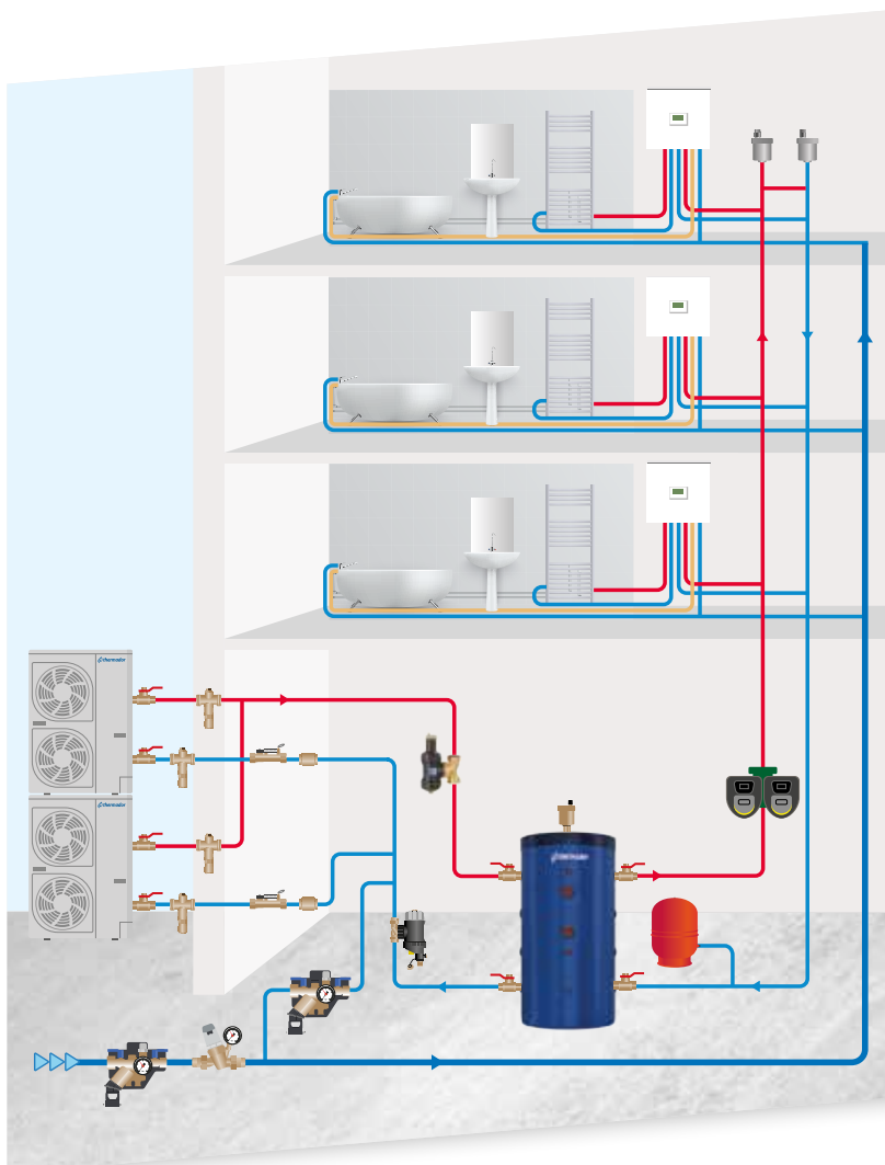
Pot de décantation CALEFFI XF
