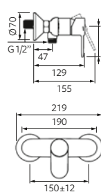
▼ Mitigeur douche
