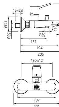
▼ Mitigeur bain/douche
