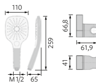
▼ Kit douchette
