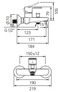
▼ Mitigeur bain/douche
