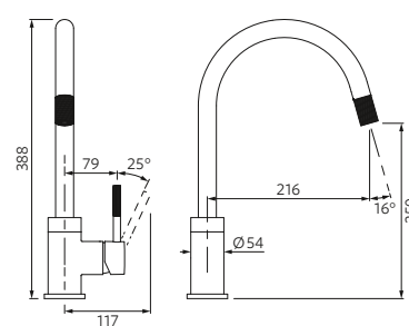
▼ Mitigeur évier
